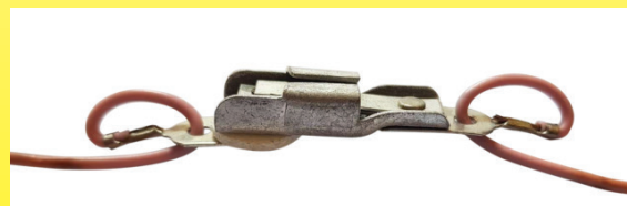
Limitador de temperatura de manta térmica de rotura lenta Calor, calibrado a 80 °C (circa 1960). Nótese la funda impermeable de PVC soldada en los cables y el bucle hecho por los conductores eléctricos que pasan por un agujero en cada terminal, esto es para eliminar tensiones de tracción en el cable (Colección Ultimheat)
