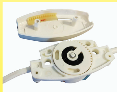
Interruptor calefactor de 3 posiciones y interruptor de apagado de 2 posiciones en manta térmica. Modelo intermedio entre sistemas rotativos y sistemas deslizantes (Circa 1970. Colección Gitem Ultiheat)
