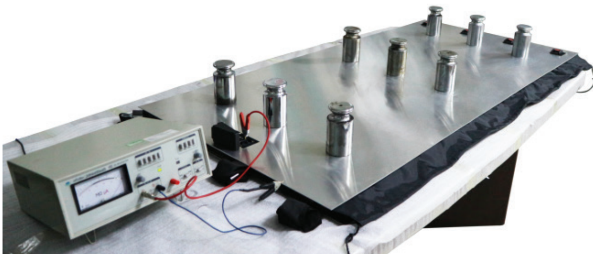
Dispositivo para medir la resistencia de aislamiento. Los valores medidos son siempre mayores a 0,1 Gohmios
